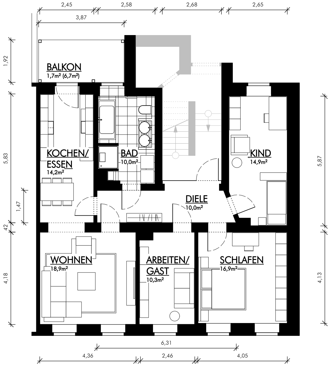
4-RAUM-WOHNUNG 97,9m 2 Goethestr. 5; 08060 Zwickau, Erdgeschoss
